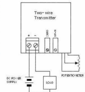
Wiring
